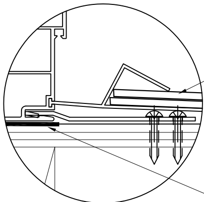
DETAIL D2A
